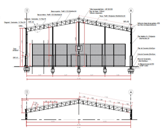
SEÇÃO DA TESOURA SE: 1.100
