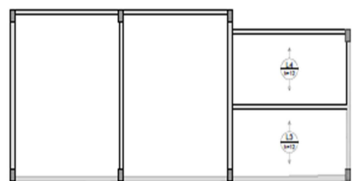
ARMATURA POSITIVA DAS LAJES DO PAVIMENTO TERREO (EIXO Y) Funda 1/10
