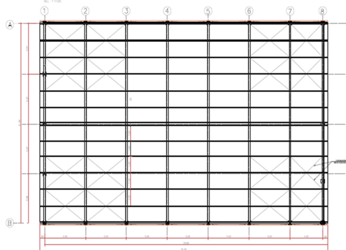
PLANTA DA ESTRUTURA DA COBERTURA
