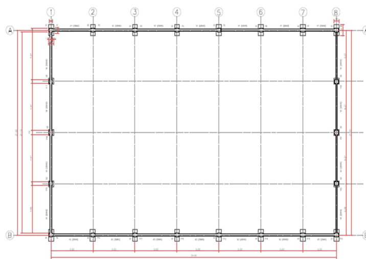
PLANTA DE LOCAÇÃO DA FUNDAÇÃO
